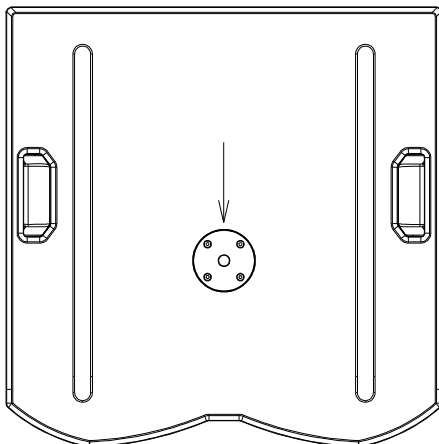
Fig. 9. S18W socket
