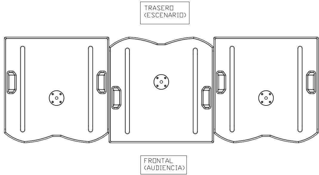
Fig. 9. Configuración cardioide básica para S18WP (horizontal en suelo)
