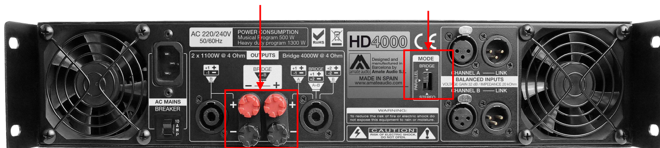
Fig. 2. Configuración S18WP
