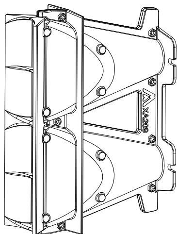
Fig. 3. Guía de ondas de altas frecuencias
