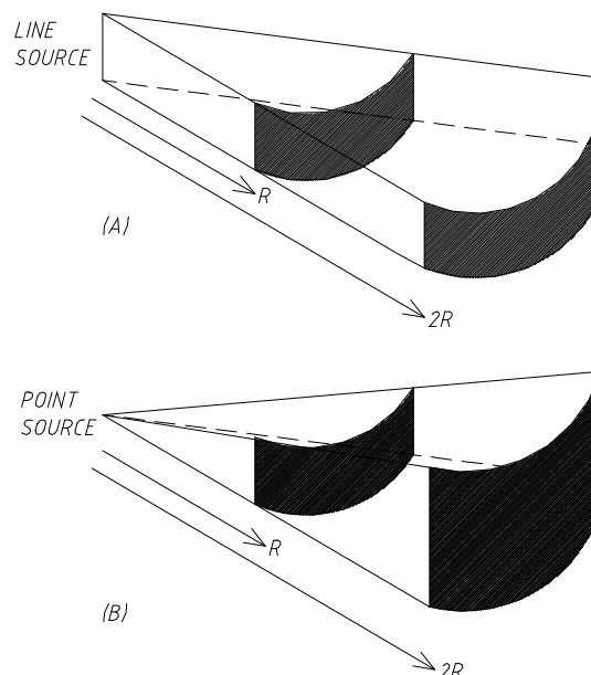
Fig. 7. Onda cilíndrica (A) vs onda esférica (B)
