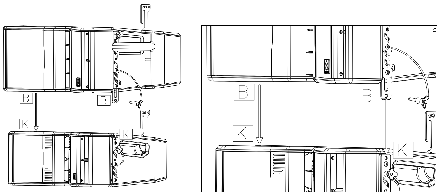
Fig. 37. Unión del recinto XA211 (superior) con XA209 (inferior). Parte frontal.
