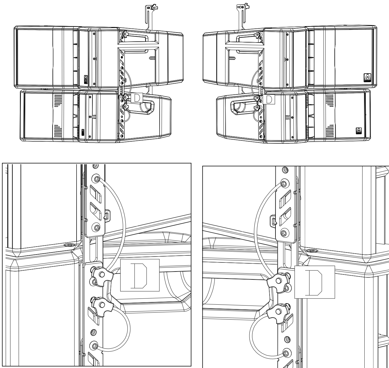
Fig. 38. Unión del recinto XA211 (superior) con XA209 (inferior) con pines pasadores
