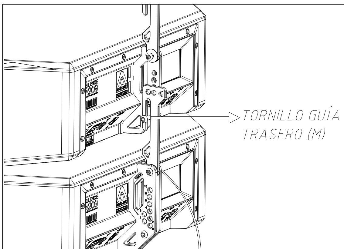
Fig. 32. Unión del recinto XA209 (superior) con XA209 (inferior). Guía rigging trasera a través de tornillo guía trasero (M).
