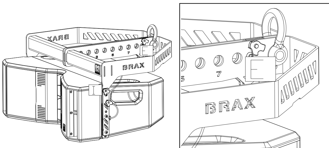
Fig. 25. Estructura de volado BRAX y recinto XA209 (primera caja). Pin trasero (E).
