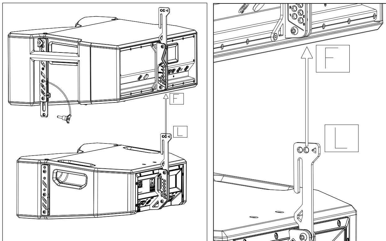
Fig. 39. Unión del recinto XA211 (superior) con XA209 (inferior). Parte trasera.
