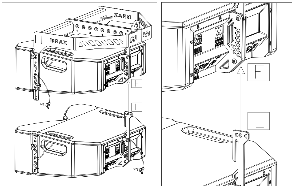
Fig. 31. Unión del recinto XA209 (superior) con XA209 (inferior). Parte trasera.
