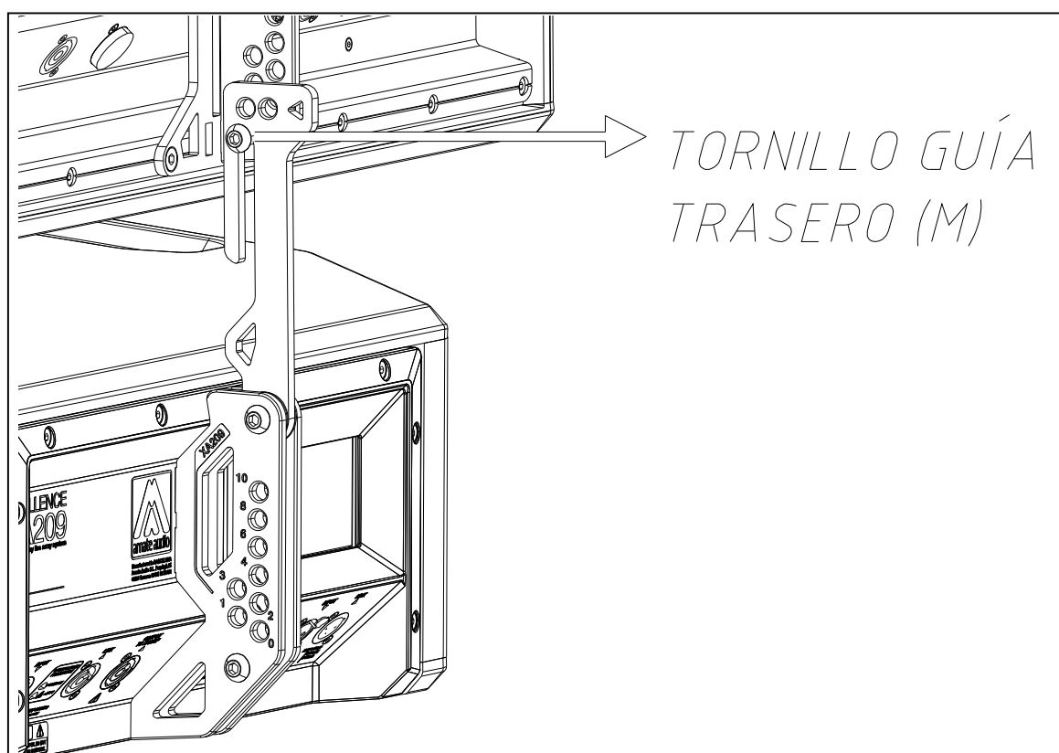
Fig. 40. Unión del recinto XA211 (superior) con XA209 (inferior). Guía rigging trasera a través de tornillo guía trasero (M).
