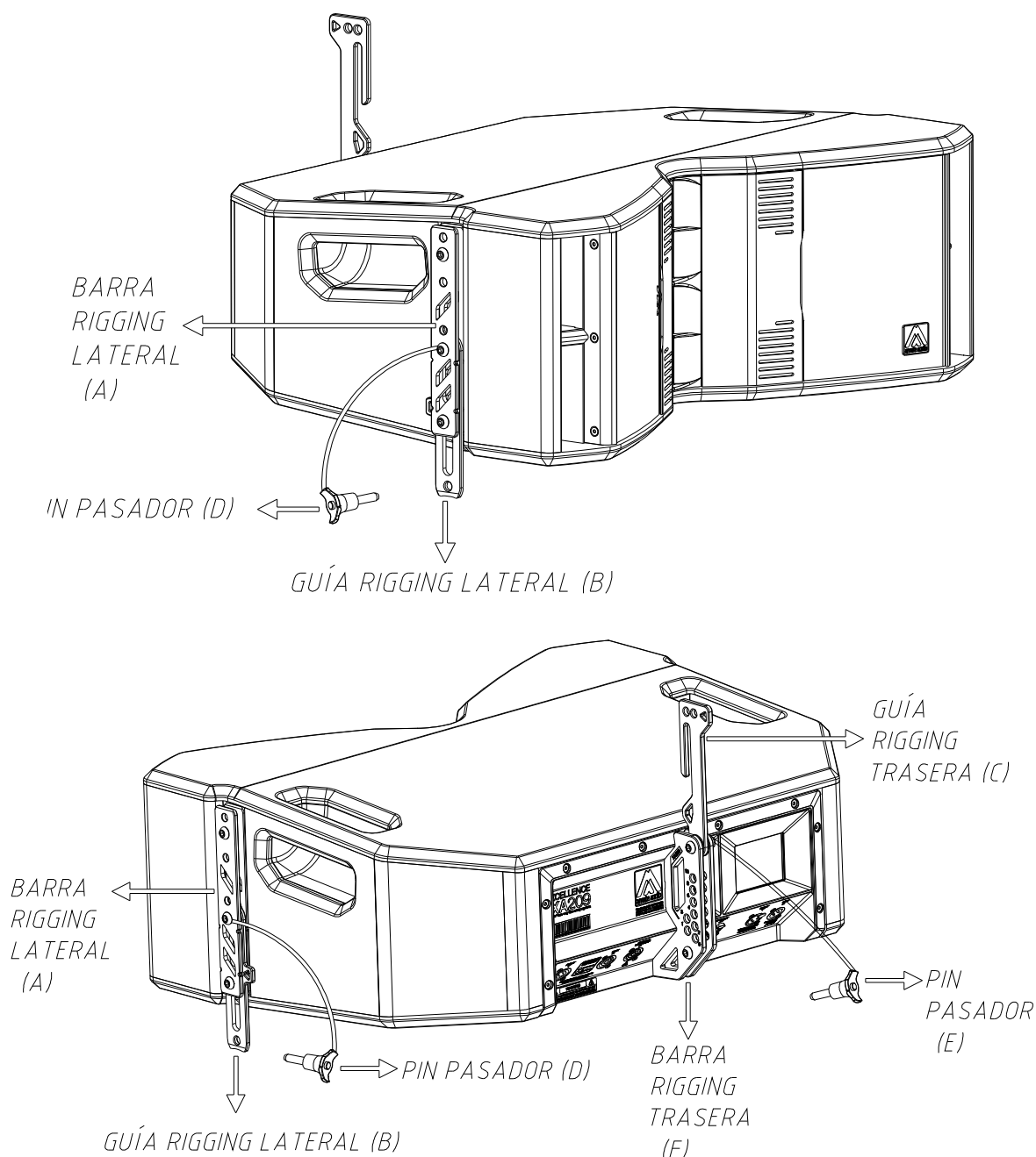
Fig. 18. Herrajes incluidos en la XA209 (laterales y trasero)
