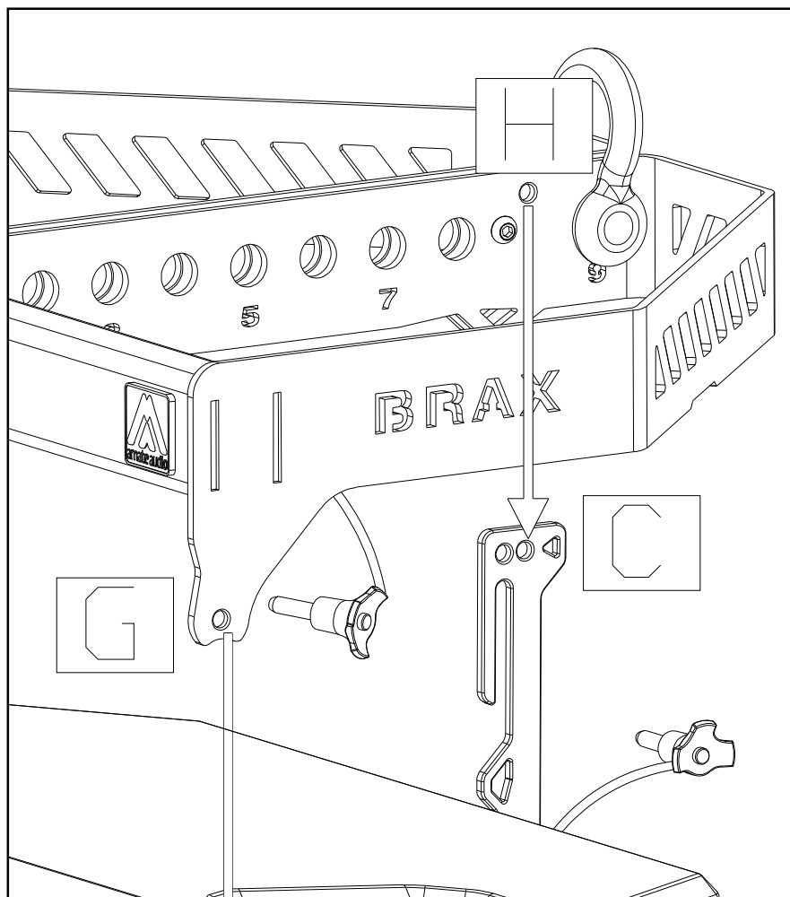
Fig. 23. Estructura de volado BRAX y recinto XA209 (primera caja)
