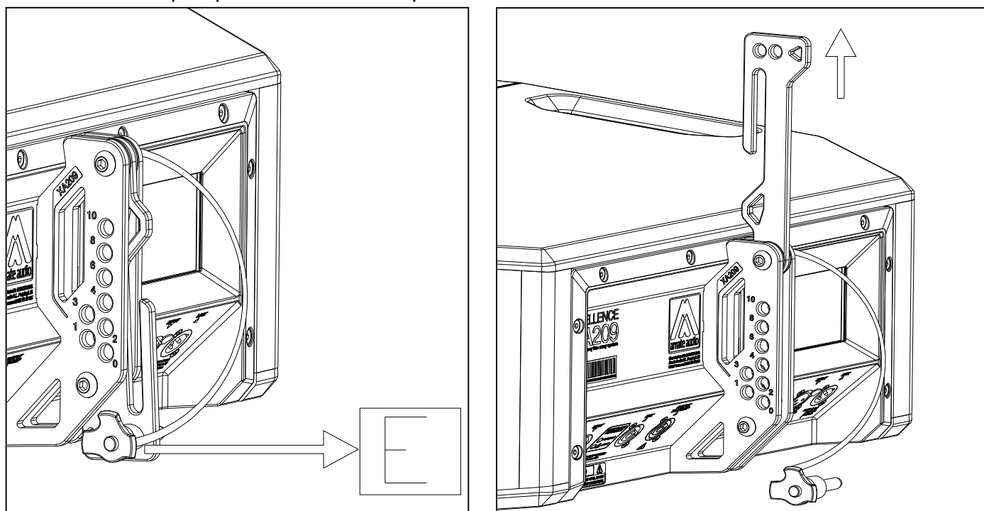
Fig. 28. Deslizamiento de la guía trasera de la XA209 (caja inferior)
