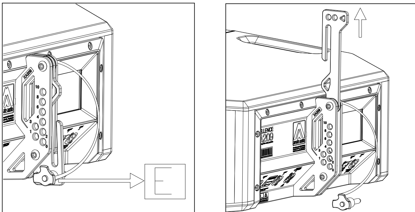
Fig. 36. Deslizamiento de la guía rigging trasera de la XA209
