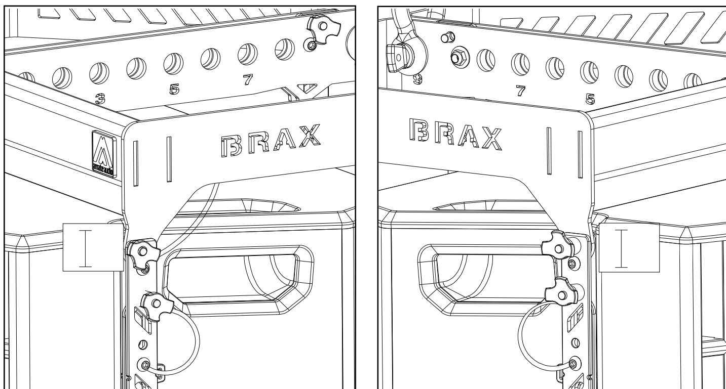
Fig. 24. Estructura de volado BRAX y recinto XA209 (primera caja). Pines delanteros (I).
