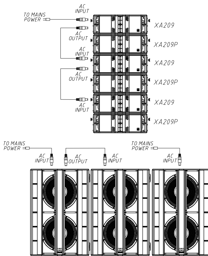
Fig. 16. Conexión eléctrica en paralelo para XA209 y XW218. Recuerde que no se pueden conectar en paralelo más de cuatro recintos del modelo XA209 ni más de dos recintos del modelo XW218 usando el conector AC Mains link.
