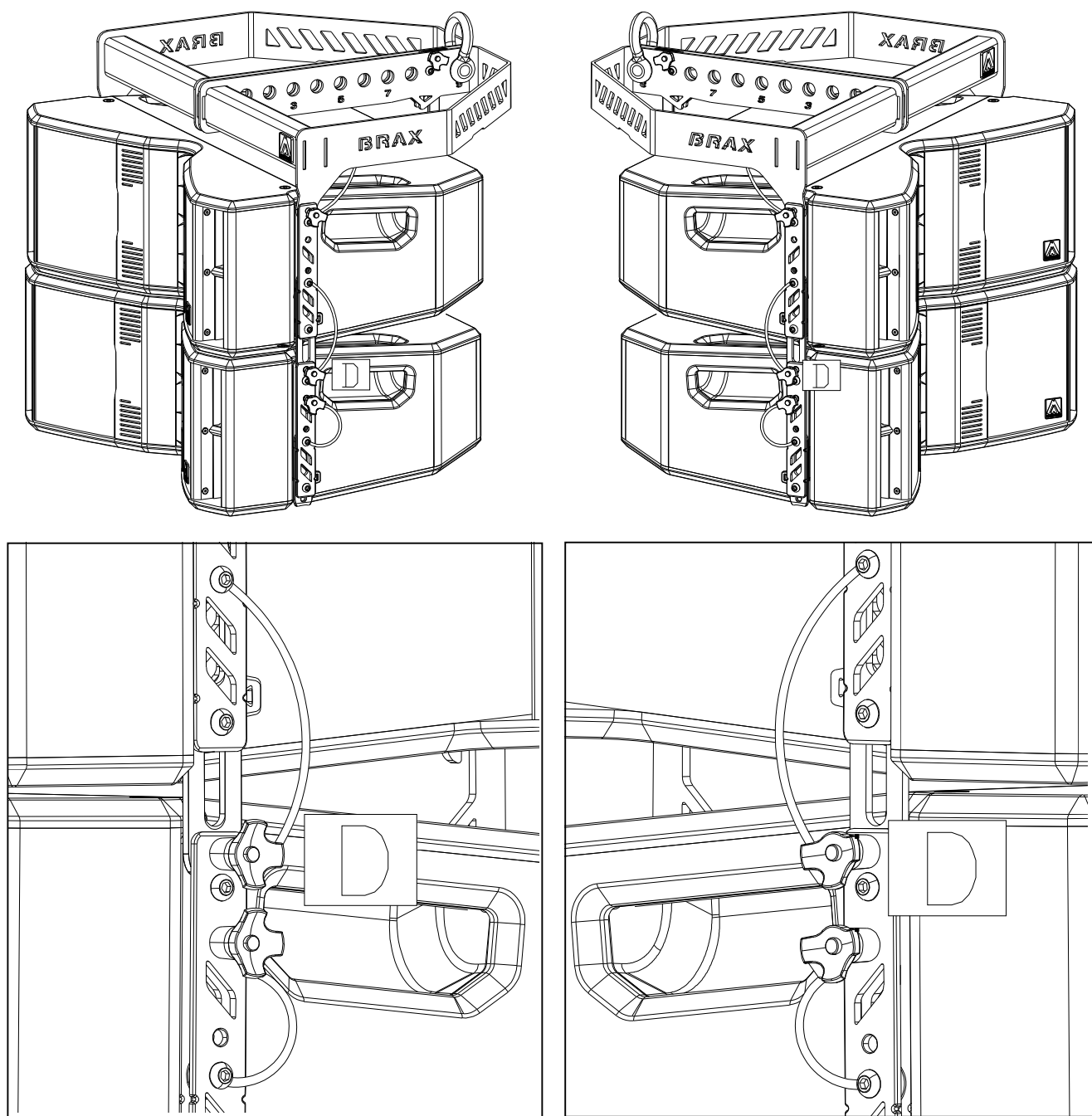
Fig. 30. Unión del recinto XA209 (superior) con XA209 (inferior) con pines pasadores
