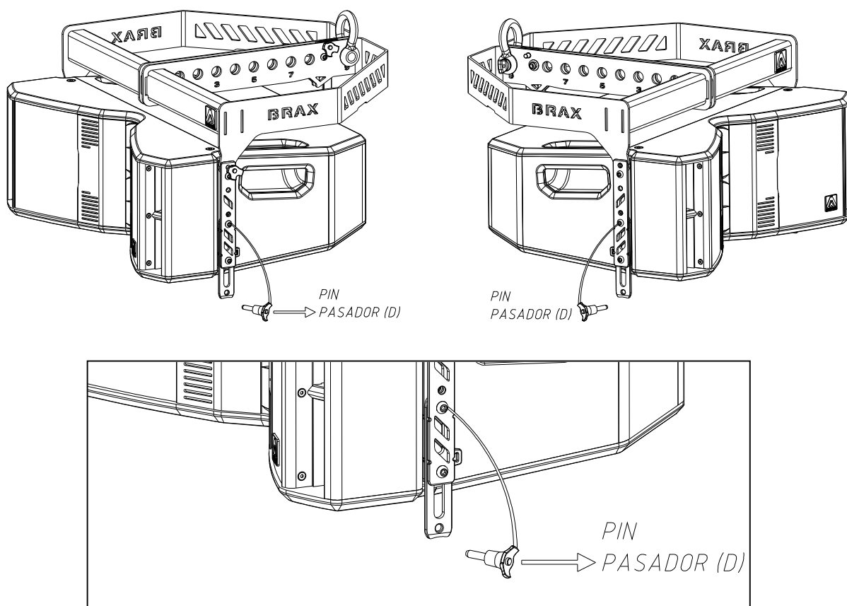
Fig. 27. Deslizamiento de las guías laterales de la XA209 (caja superior)
