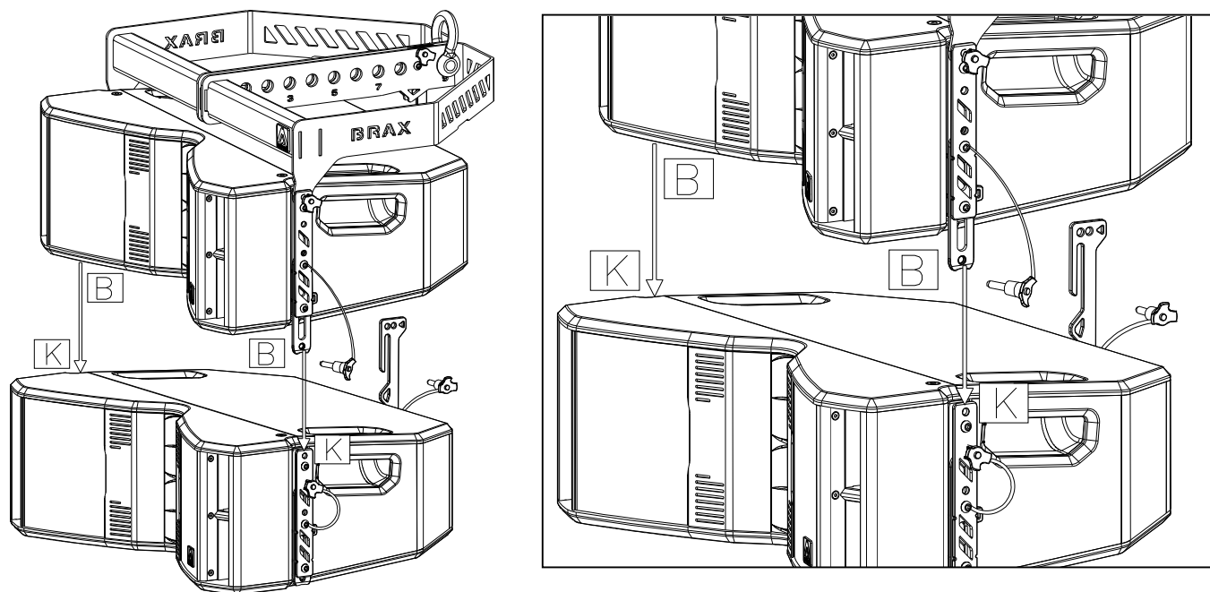
Fig. 29. Unión del recinto XA209 (superior) con XA209 (inferior). Parte frontal.
