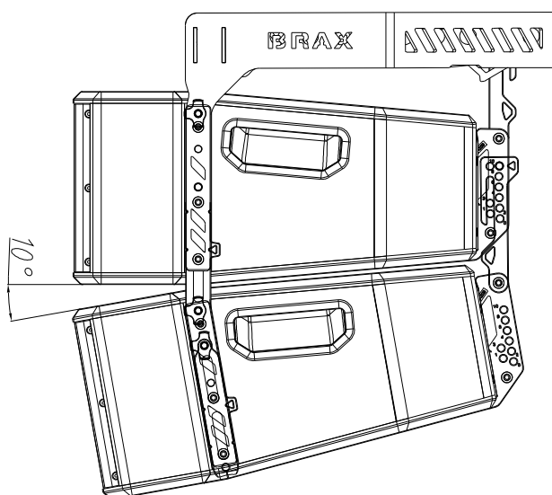
Fig. 4. Inclinación entre cajas (máximo 10°)
