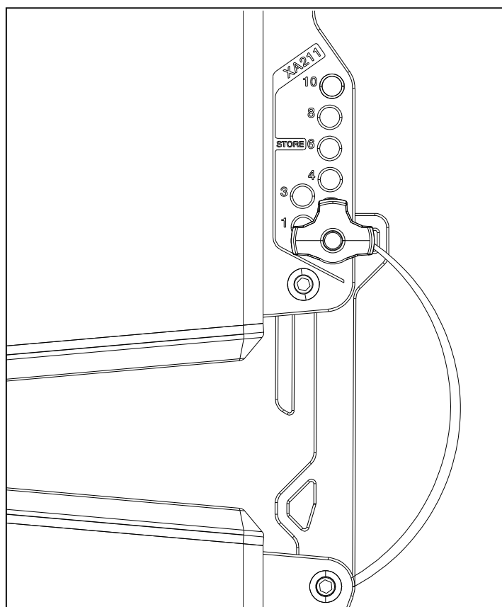
Fig. 42. Coloque en la XA211 el pin pasador trasero de la XA209
