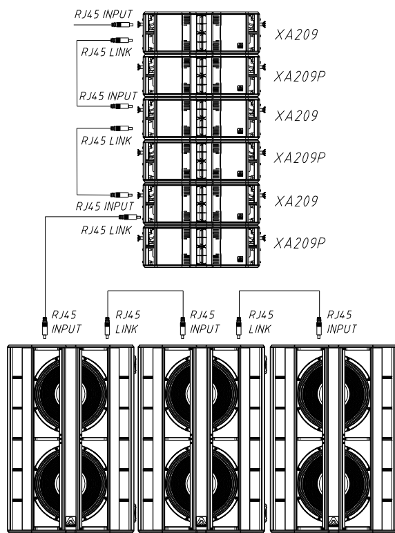
Fig. 17. Conexión red Ethernet para XA209 y XW218. No encadenar más de ocho unidades de XA209 o de XW218 tal y como se muestra en la figura.
