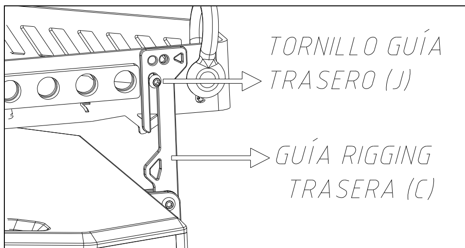
Fig. 26. Estructura de volado BRAX y recinto XA209 (primera caja). Guía rigging trasera (C) a través de tornillo guía trasero (J).
