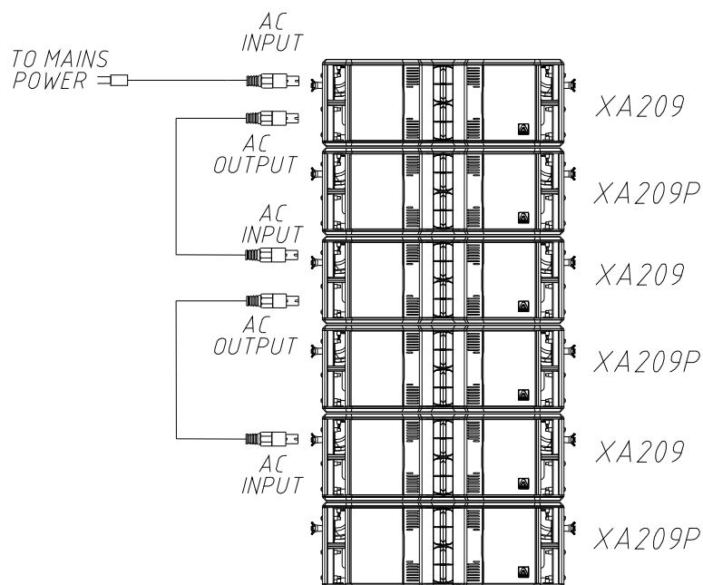
Fig. 13. Conexión en paralelo para XA209 (Red). Máximo cuatro unidades linkadas
