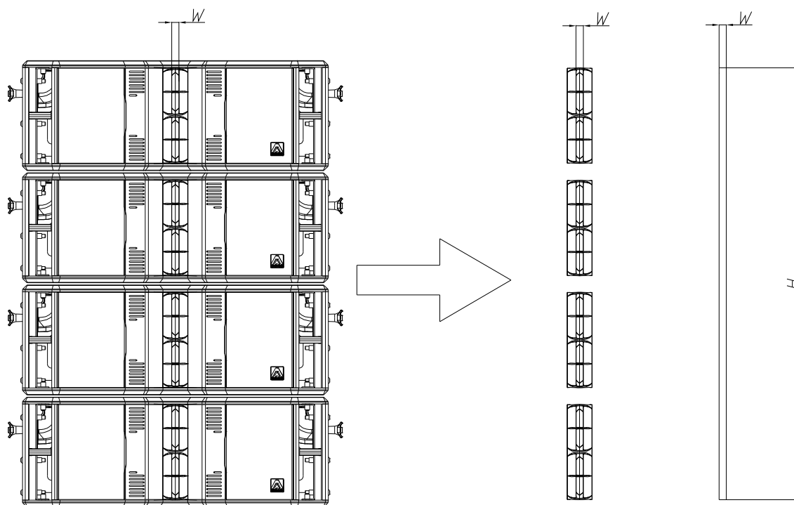
Fig. 2. Segundo criterio de "arrayabilidad"
