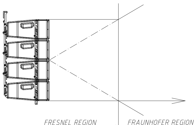
Fig. 5. Límites zona Fresnel-Fraunhofer
