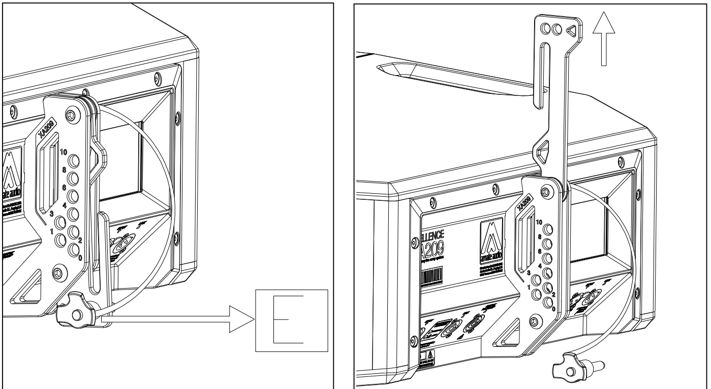
Fig. 22. Deslizamiento de la guía rigging trasera de la XA209 (primera caja)
