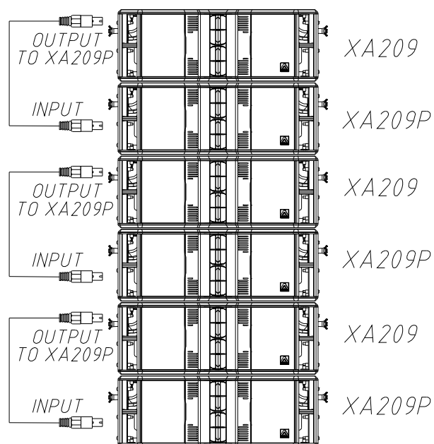
Fig. 14. Conexión entre unidades XA209 (activas) y XA209P (pasivas)
